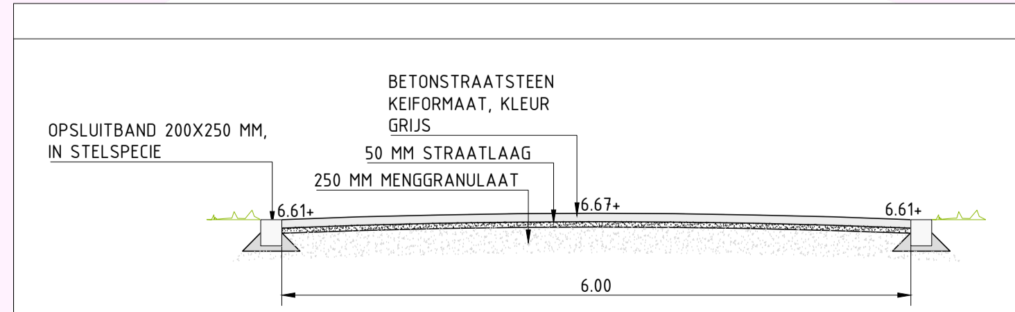
DWARSPROFIEL PLATEAU SCHAAL 1:50
