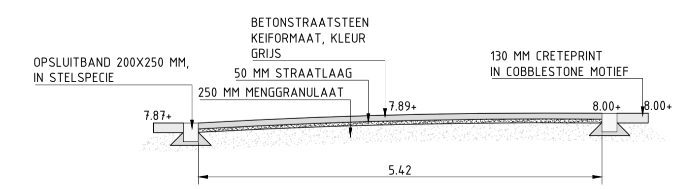
DWARSPROFIEL PLATEAU SCHAAL 1:50
