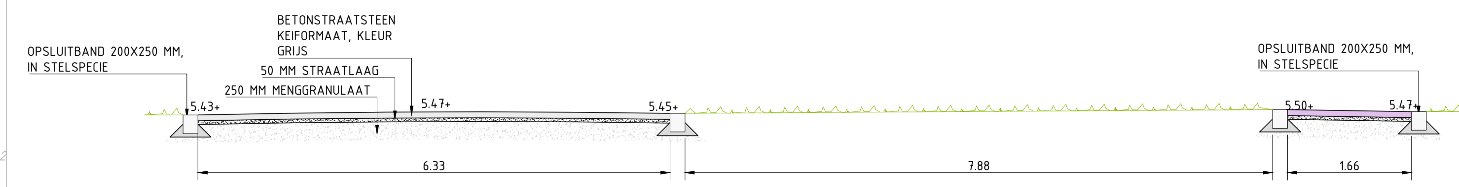
DWARSPROFIEL PLATEAU SCHAAL 1:50
