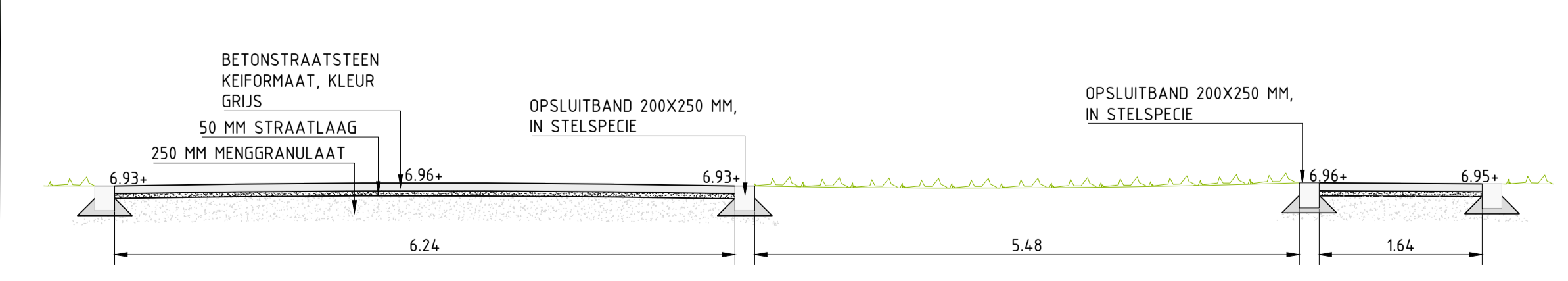
DWARSPROFIEL PLATEAU SCHAAL 1:50
