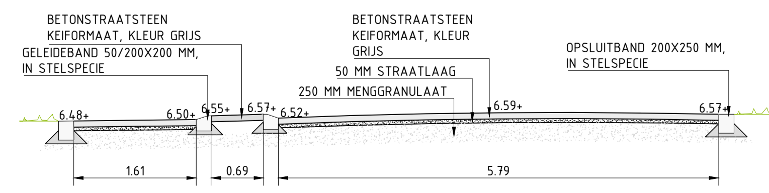
DWARSPROFIEL PLATEAU SCHAAL 1:50
