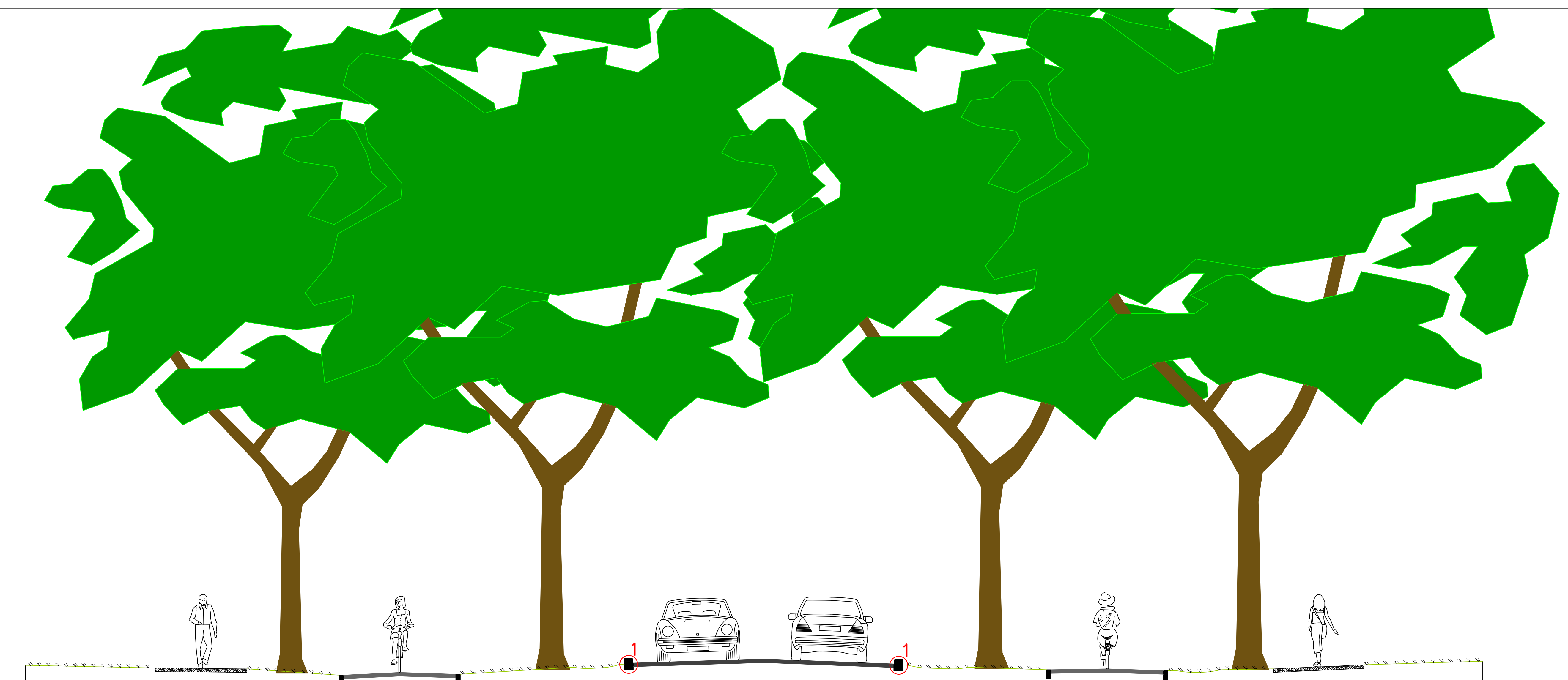
Profiel A-A Schaal 1:50
