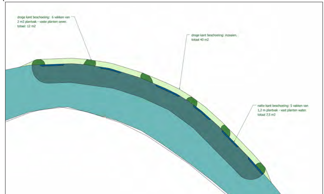
Ecozone 3c: uitwerking plantvakken en in te zaaien zone
