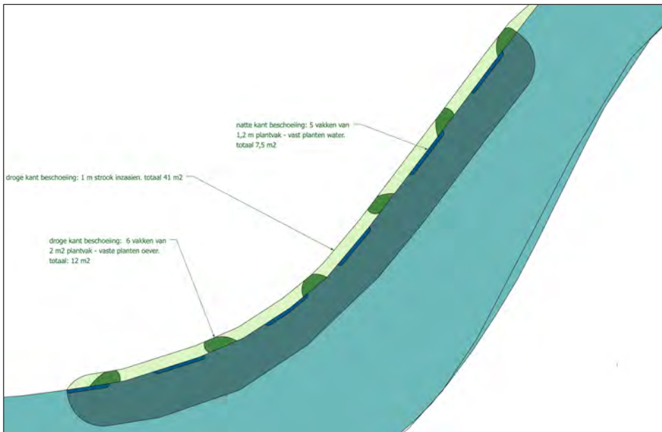
Ecozone 3a: uitwerking plantvakken en in te zaaien zone
